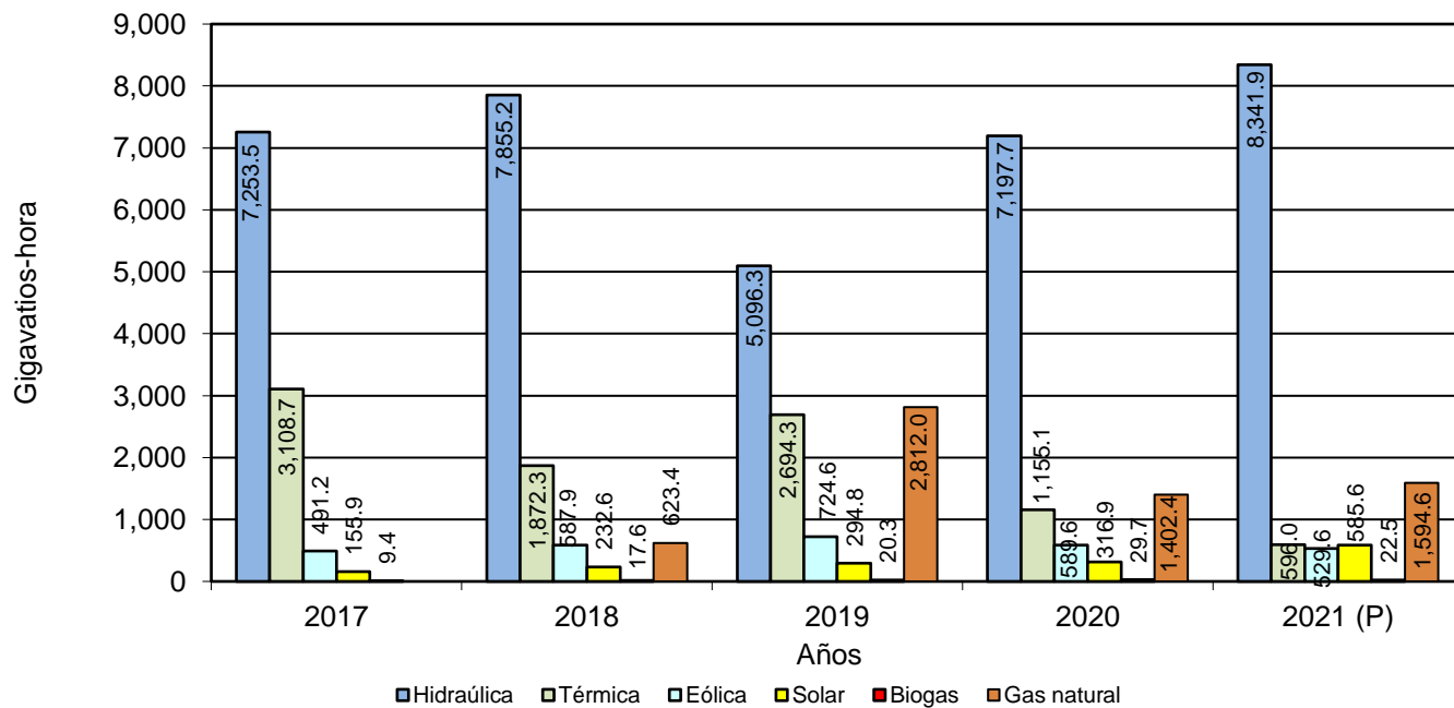
GENERACIÓN BRUTA DE ELECTRICIDAD EN LA REPÚBLICA: AÑOS 2017-21
