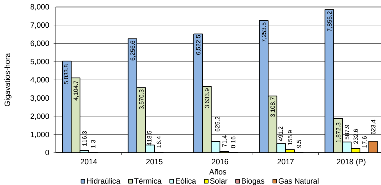
GENERACIÓN BRUTA DE ELECTRICIDAD EN LA REPÚBLICA: AÑOS 2014-18
