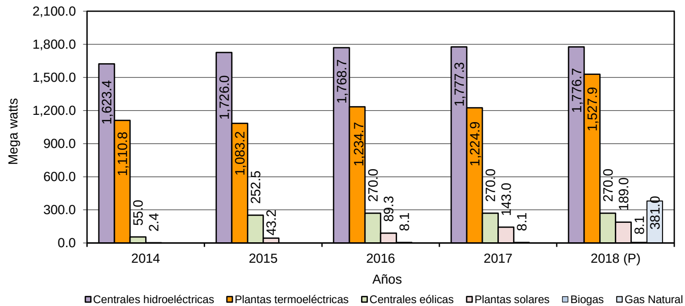
CAPACIDAD INSTALADA DE GENERACIÓN ELÉCTRICA EN LA REPÚBLICA: AÑOS 2014-18
