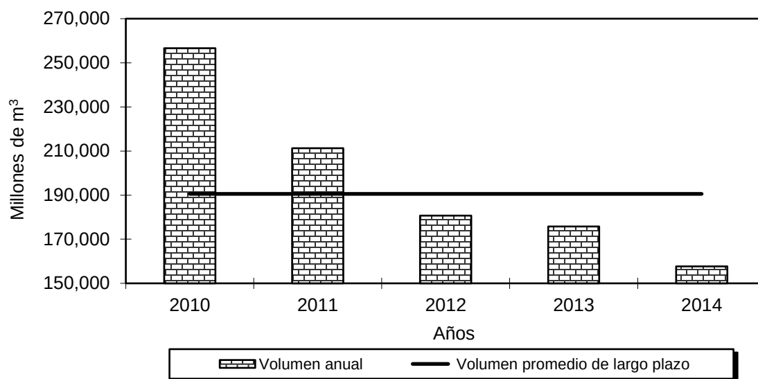
ESTIMACIÓN DEL VOLUMEN DE AGUA PROVENIENTE DE LA PRECIPITACIÓN EN LA REPÚBLICA: AÑOS 2010-14
