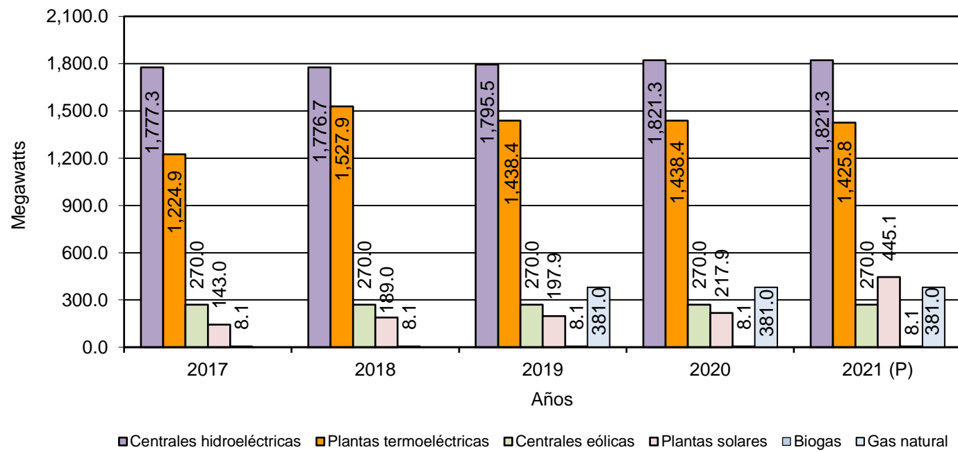
CAPACIDAD INSTALADA DE GENERACIÓN ELÉCTRICA EN LA REPÚBLICA: AÑOS 2017-21
