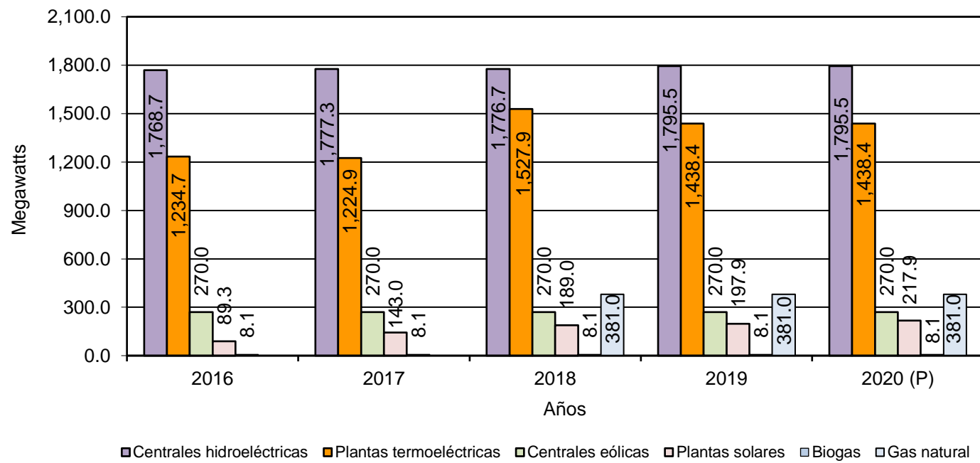
CAPACIDAD INSTALADA DE GENERACIÓN ELÉCTRICA EN LA REPÚBLICA: AÑOS 2016-20
