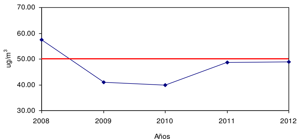
CONCENTRACIONES PROMEDIO DE PM-10 REGISTRADAS EN LA ESTACIÓN DE LA UNIVERSIDAD DE PANAMÁ: AÑOS 2008-12
