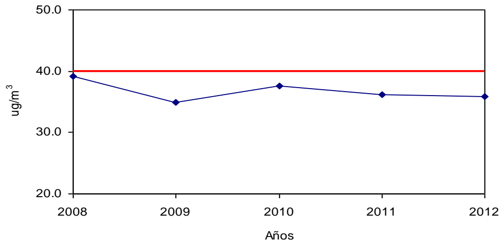
CONCENTRACIONES PROMEDIO DE NOx REGISTRADAS EN LA ESTACIÓN DE LA UNIVERSIDAD DE PANAMÁ: AÑOS 2008-12
