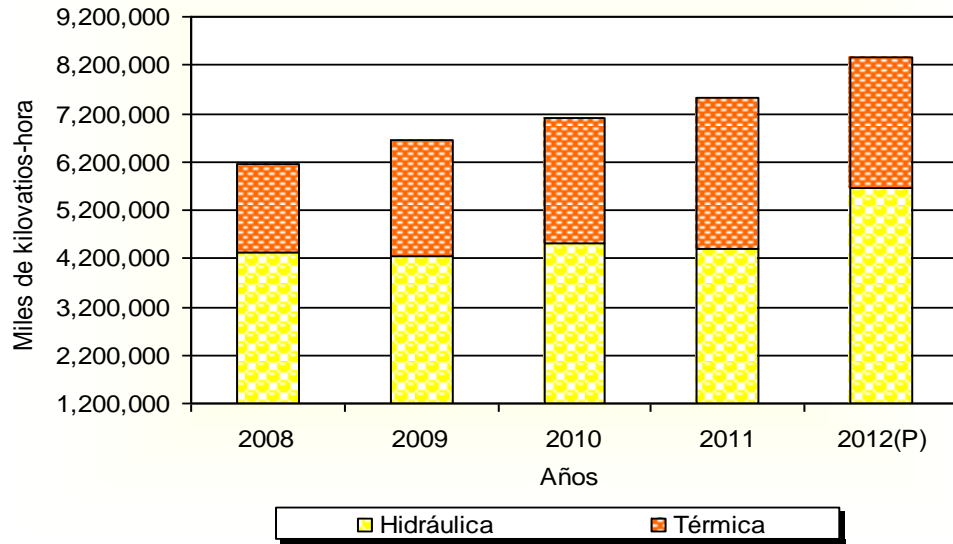
GENERACIÓN BRUTA DE ELECTRICIDAD EN LA REPÚBLICA, POR TIPO DE GENERADORA: AÑOS 2008-12
