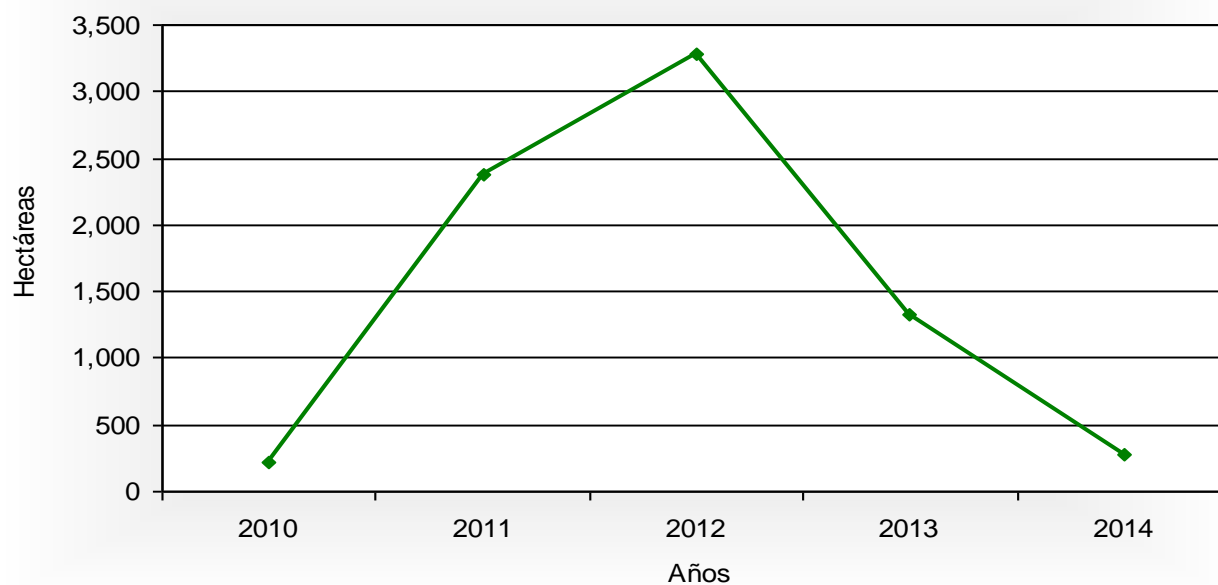
SUPERFICIE REFORESTADA EN LA REPÚBLICA: AÑOS 2010-14
