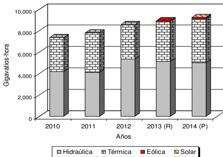
GENERACIÓN BRUTA DE ELECTRICIDAD EN EL SISTEMA INTERCONECTADO NACIONAL: AÑOS 2010-14
