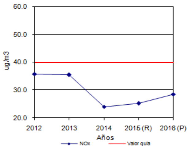
CONCENTRACIÓN PROMEDIO DE NOx REGISTRADA EN LA ESTACIÓN DE LA UNIVERSIDAD DE PANAMÁ: AÑOS 2012-16
