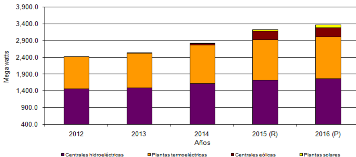
CAPACIDAD INSTALADA DE GENERACIÓN ELÉCTRICA EN LA REPÚBLICA: AÑOS 2012-16
