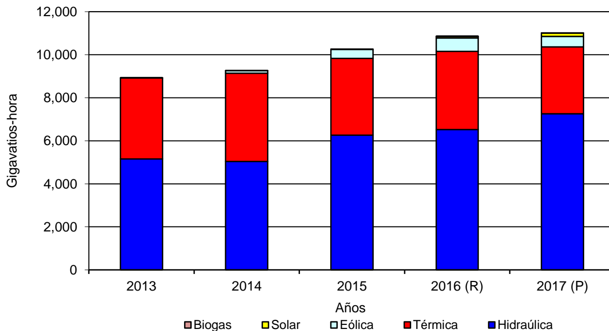
GENERACIÓN BRUTA DE ELECTRICIDAD EN LA REPÚBLICA: AÑOS 2013-17
