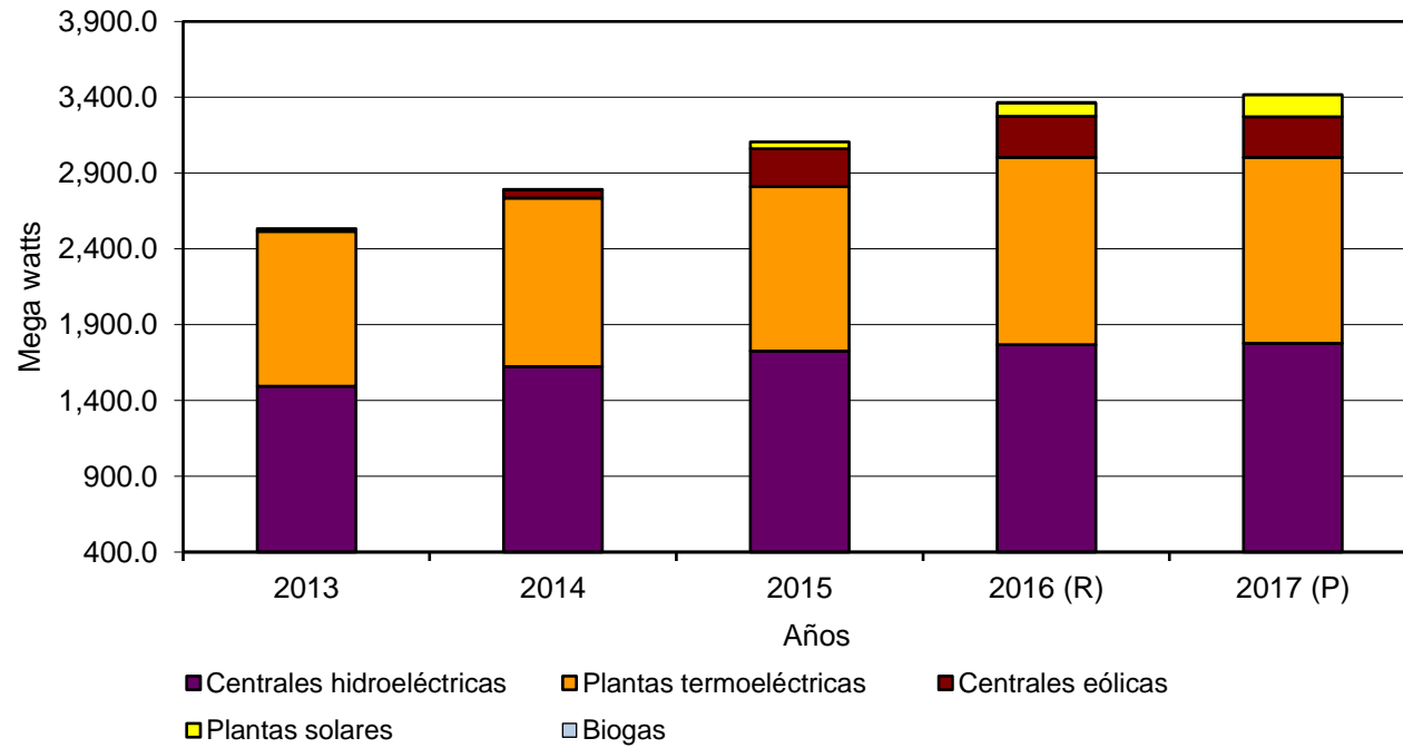
CAPACIDAD INSTALADA DE GENERACIÓN ELÉCTRICA EN LA REPÚBLICA: AÑOS 2013-17
