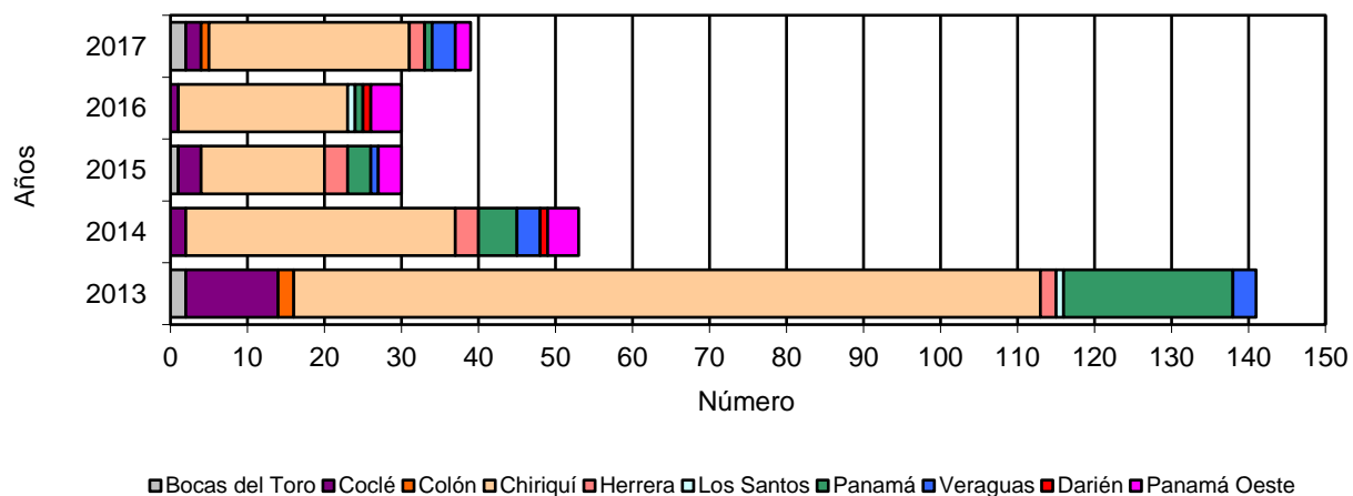
CONCESIONES DE AGUA EN LA REPÚBLICA: AÑOS 2013-17
